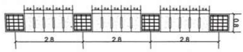
DRAINAGE LAYOUT SCALE: 1:100
