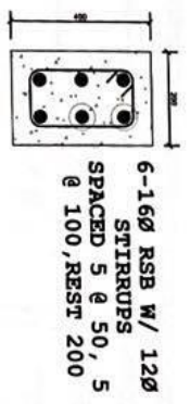
TB-1/B-1 DETAILS SCALE:
