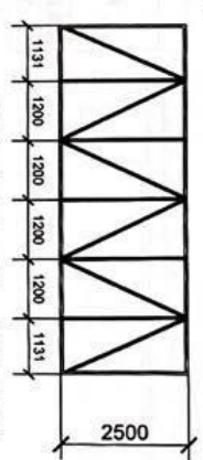
TR-2 PLAN SCALE:
